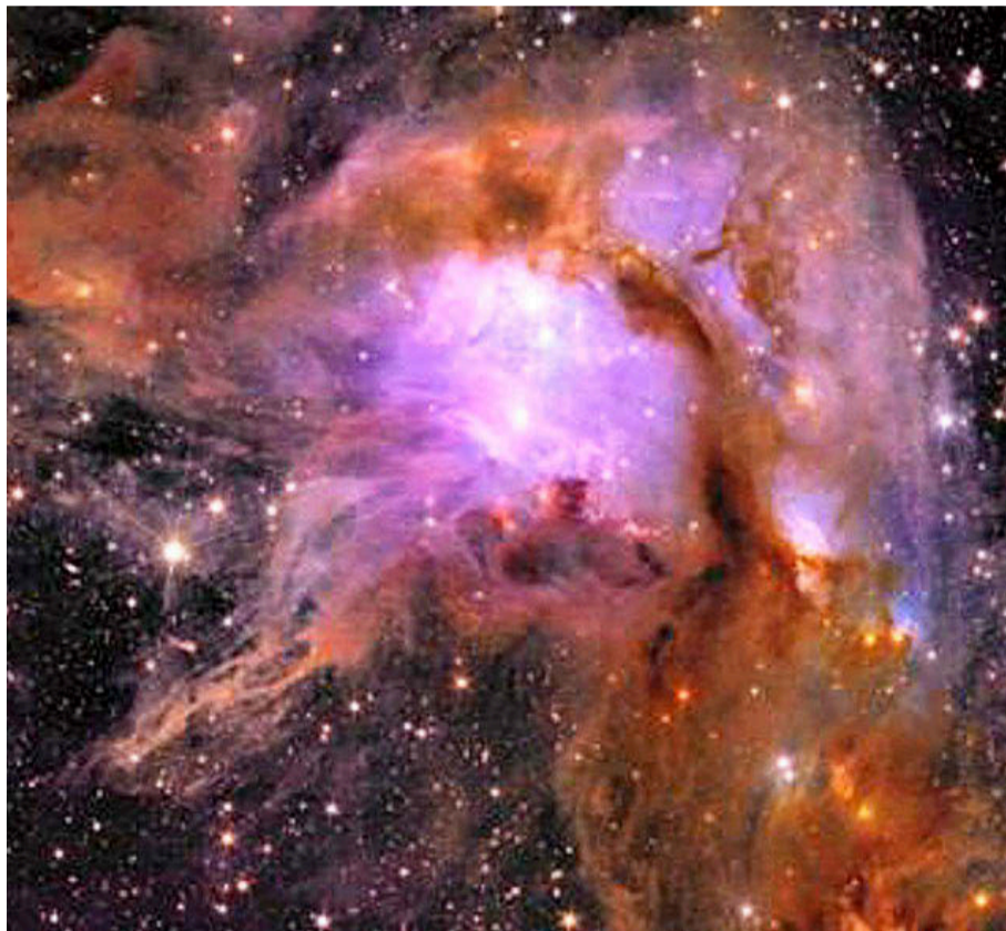
Nueva imagen de la región de formación estelar Messier 78.
