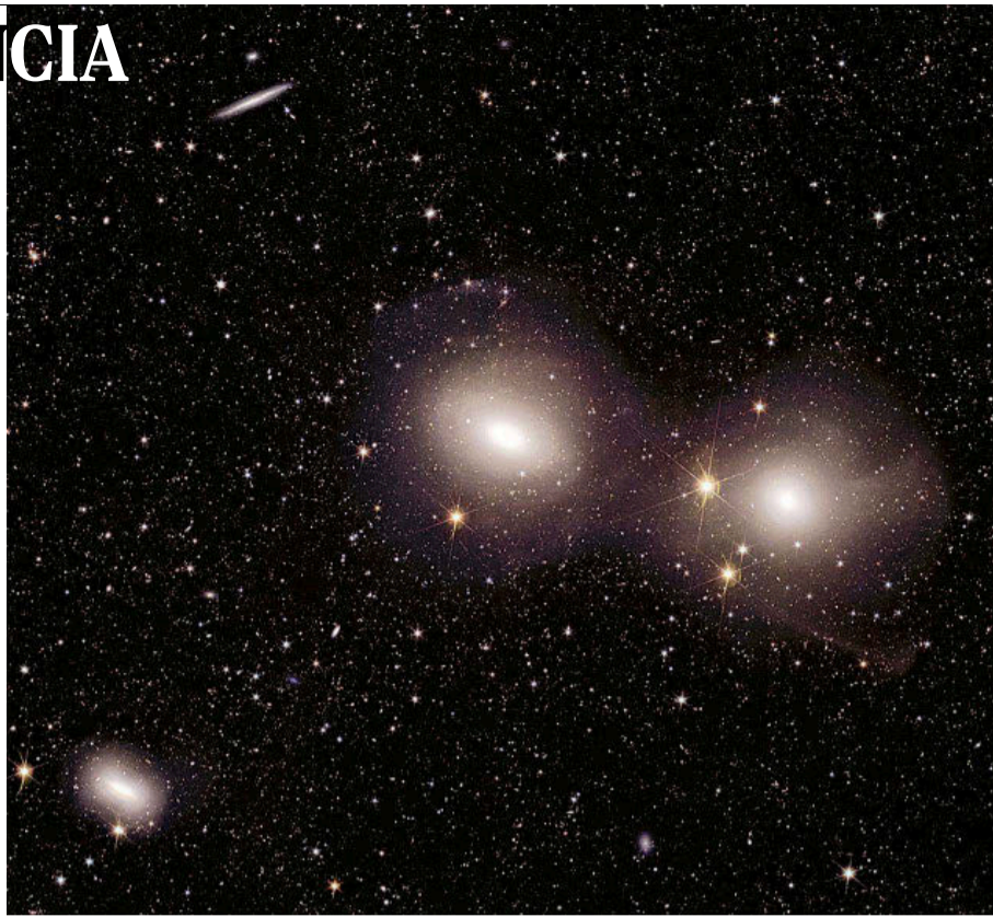
Tres imágenes captadas por la nave 'Euclid'. A la izquierda, el grupo de galaxias del Dorado.
