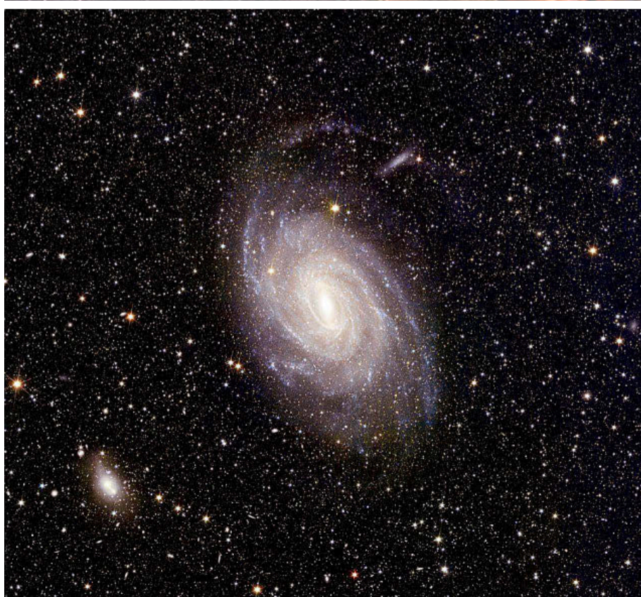
La galaxia espiral NGC 6744. FOTOS: ESA/CONSORCIO EUCLID/NASA
